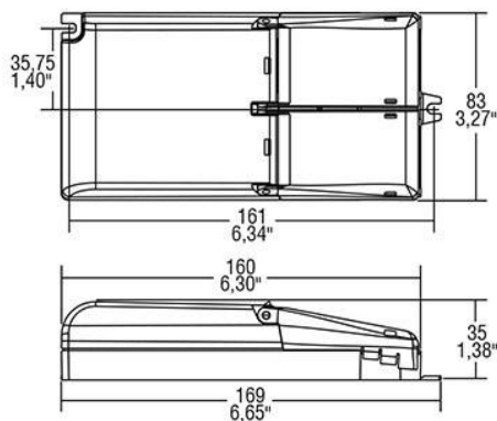
Maßzeichnung
