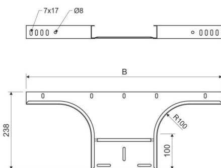
Maßzeichnung
