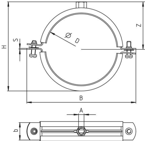
Strichzeichnung
