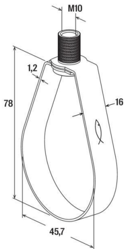
Maßzeichnung
