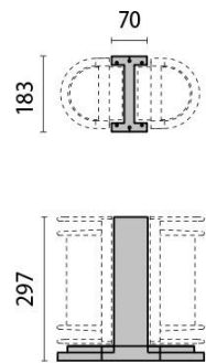
Maßzeichnung
