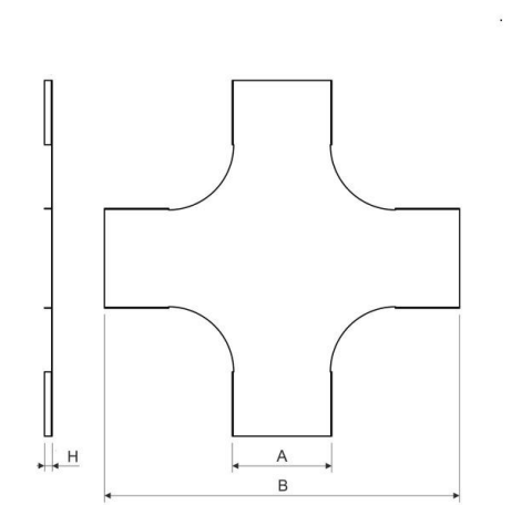
Maßzeichnung
