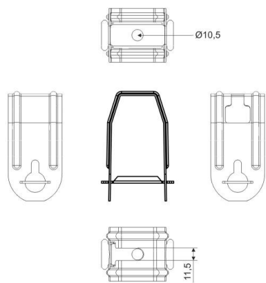
Maßzeichnung
