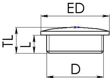
Maßzeichnung
