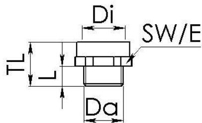
Maßzeichnung
