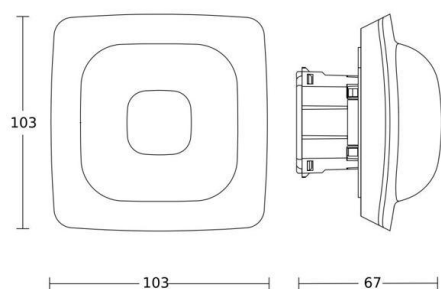
Maßzeichnung
