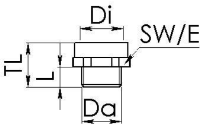
Maßzeichnung
