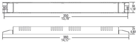
Maßzeichnung
