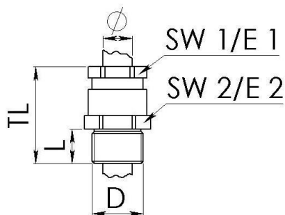
Maßzeichnung
