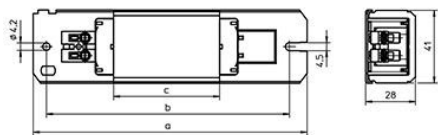
Maßzeichnung
