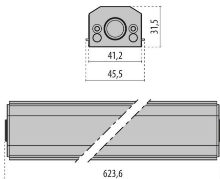
Maßzeichnung
