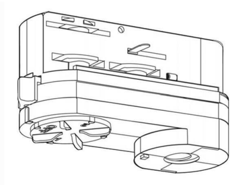
Multiadapter XTSA68-3, weiss, Tragkraft max.10kg
