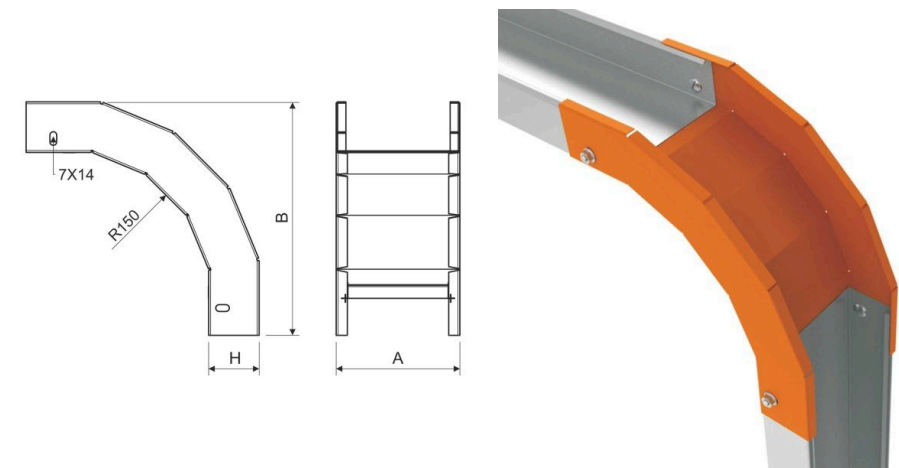
Maßzeichnung
