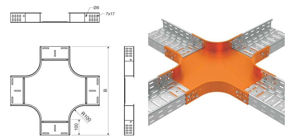
Maßzeichnung
