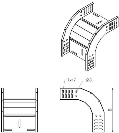
Maßzeichnung
