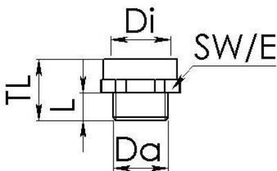
Maßzeichnung
