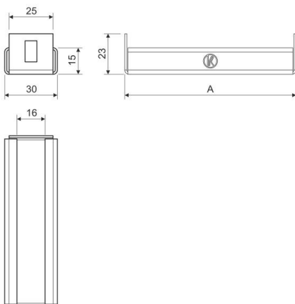
Maßzeichnung
