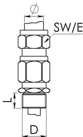
Maßzeichnung
