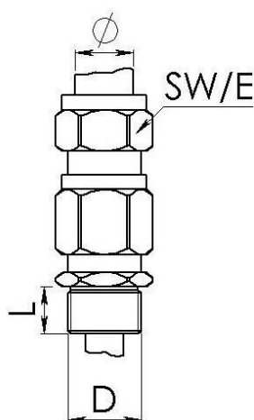
Maßzeichnung
