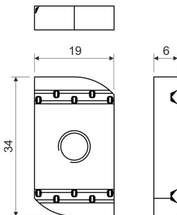
Maßzeichnung
