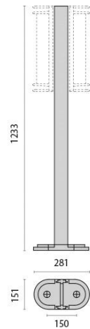
Maßzeichnung
