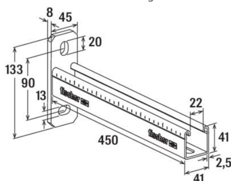
Maßzeichnung
