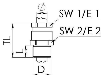
Maßzeichnung
