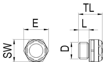
Maßzeichnung
