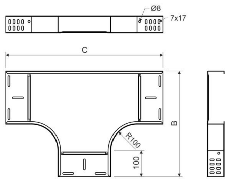
Maßzeichnung
