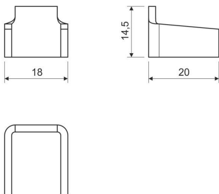
Maßzeichnung
