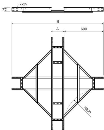
Maßzeichnung
