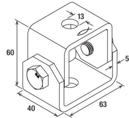
Maßzeichnung
