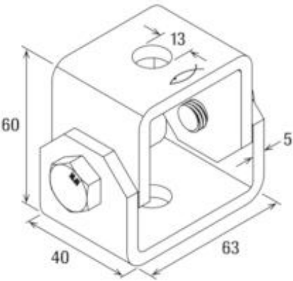
Strichzeichnung
