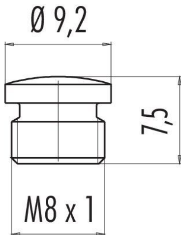
Maßzeichnung
