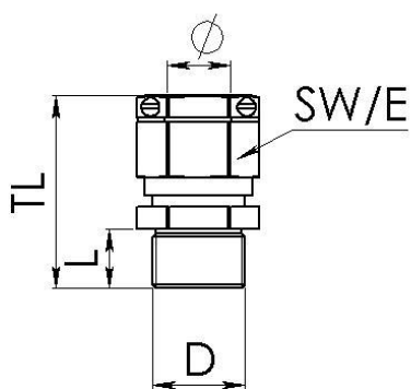
Maßzeichnung
