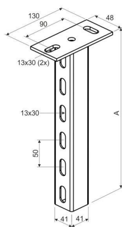
Maßzeichnung
