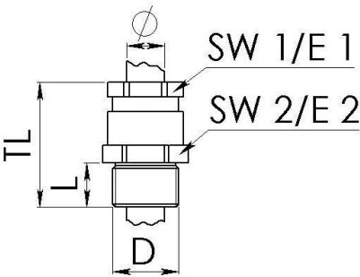
Maßzeichnung
