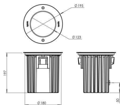
Maßzeichnung
