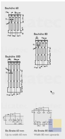
Maßzeichnung
