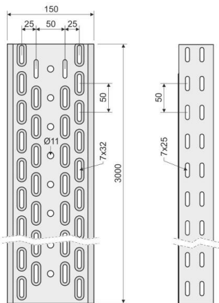
Maßzeichnung
