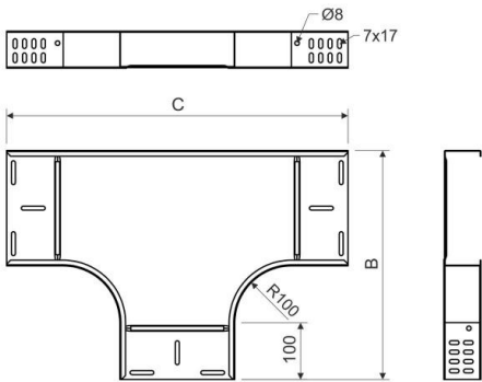
Maßzeichnung
