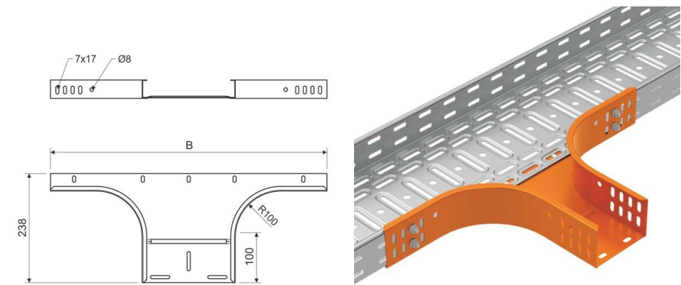
Maßzeichnung
