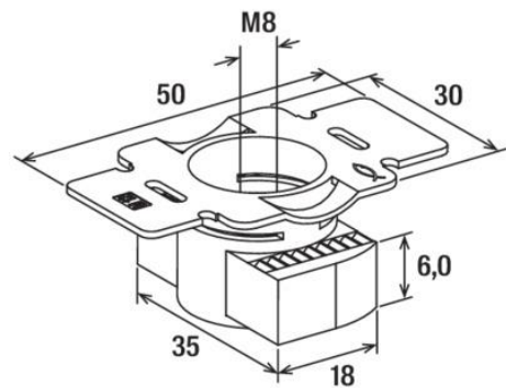
Maßzeichnung
