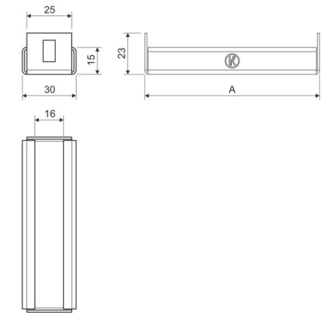
Maßzeichnung
