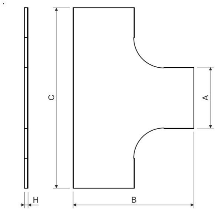
Maßzeichnung
