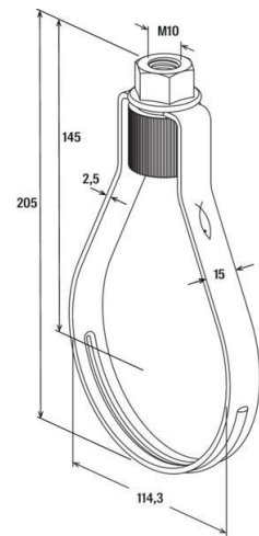
Maßzeichnung
