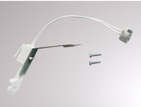
Fassung GU5,3 mit Klemme & Zugentlastung
