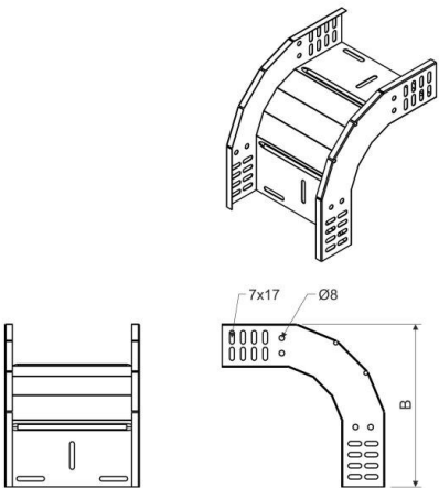
Maßzeichnung
