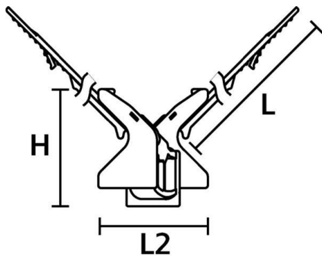
Maßzeichnung
