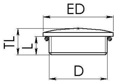
Maßzeichnung
