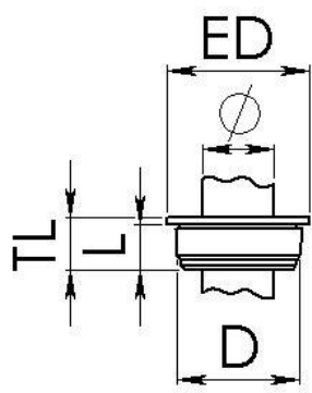
Maßzeichnung
